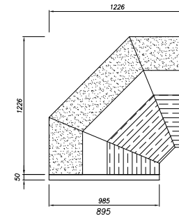
ANGOLO INTERNO 90° DIAGONALE
