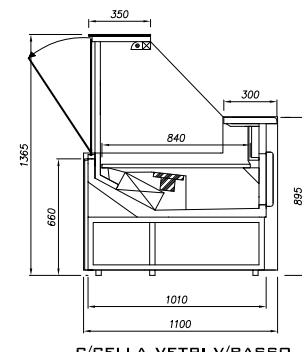
C/CELLA VETRI V/BASSO
