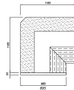
ANGOLO INTERNO 90° SQUADRATO
