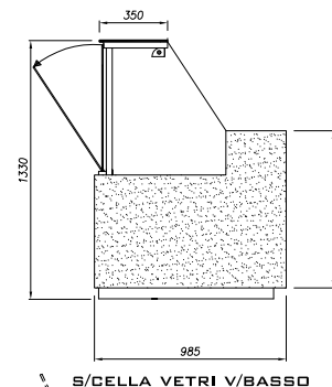
S/CELLA VETRI V/BASSO
